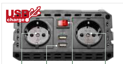
Schuko USB: 5V-3,1A On / Off Schuko
