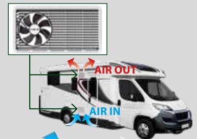
Ventola di raffreddamento Collegamento cavi
